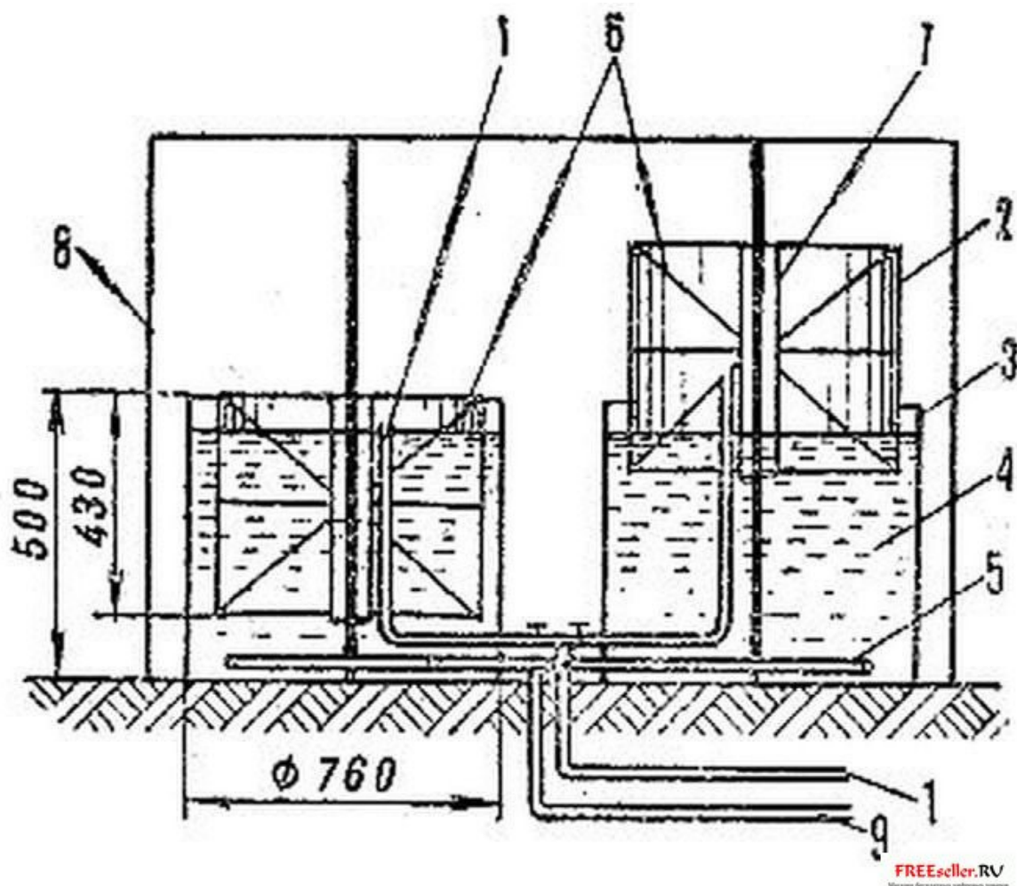
Рис. 3 Схема установки для получения биогаза повышенной производительности
