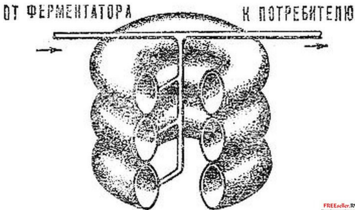
Рис. 2 Разбухающий рещервуар из тракторных камер
