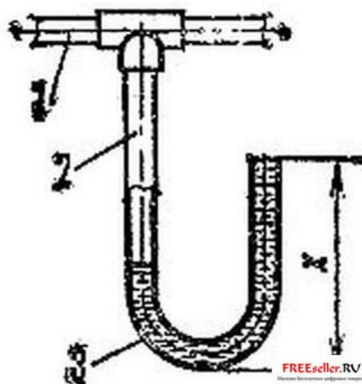
Рис. 4 Схема устройства для отвода конденсированной воды
